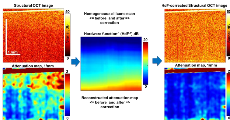
Рис. 1. Карта корректирующей функции, ОКТ-сканы однородного образца и соответствующие им карты коэффициента затухания до и после коррекции.
