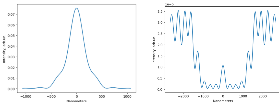
Рис. 1. Распределение интенсивности в фокальной плоскости при фокусировке радиально поляризованной моды R-TEM 01 с параметром \beta = 1 (а) и при фокусировке радиально поляризованного пучка Бесселя-Гаусса, прошедшего через бинарную фазовую маску, состоящую из 108 зон (б) апланатическим объективом с числовой апертурой равной 0,95
