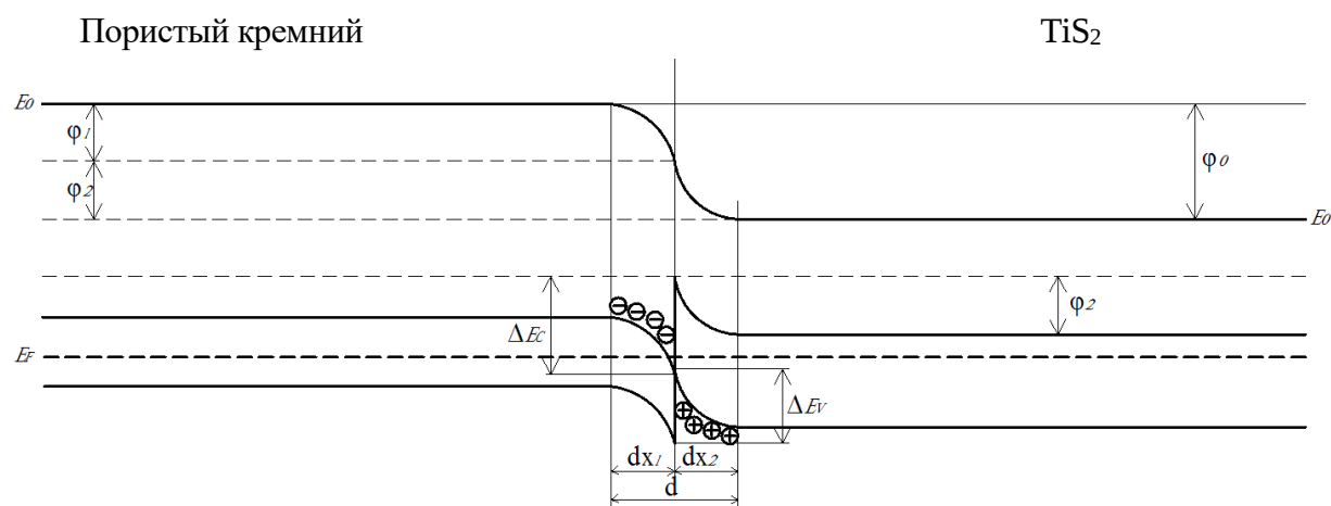
Рис. 2. Энергетическая диаграмма гетероперехода P-Si– \text{TiS}_2
