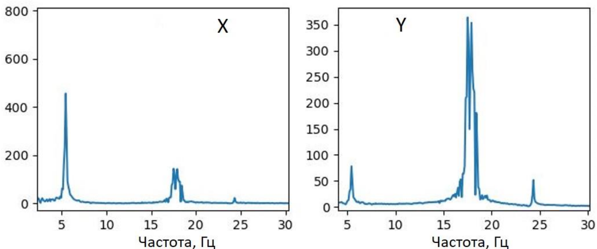
Рис. 3. Частоты горизонтальных (X) и вертикальных (Y) осцилляций центра левитируемой капли
