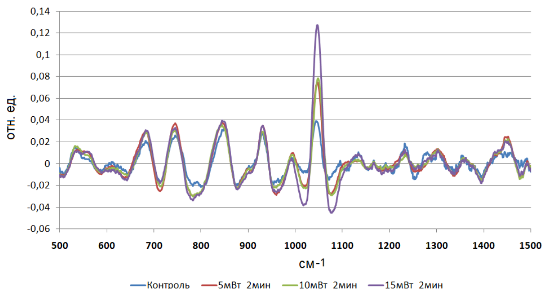
Рис. 1. Спектры для контрольного образца и образцов, облученных с мощностью 5, 10 и 15 мВт в течение 2 минут
