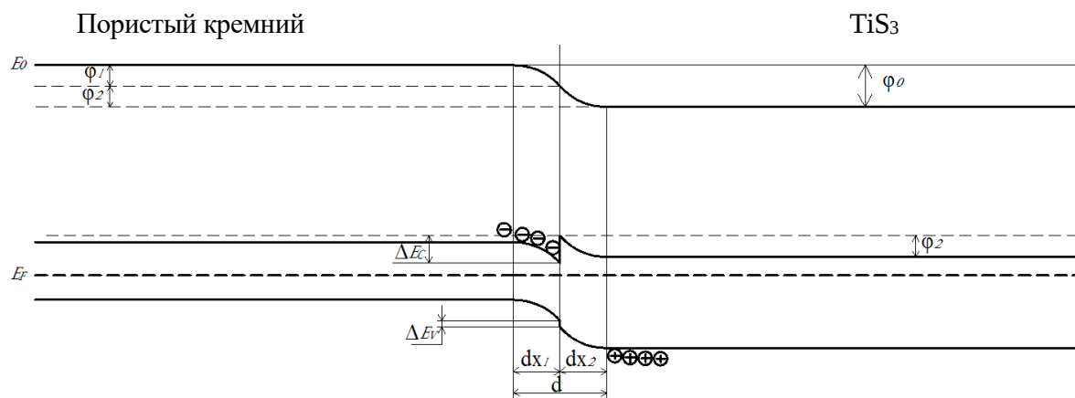
Рис. 1. Энергетическая диаграмма гетероперехода P-Si– \text{TiS}_3
