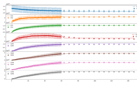
Рис. 2 - Временные эволюции ИК-Фурье линий для продуктов радиационно-инициируемых реакций в метановом льду
