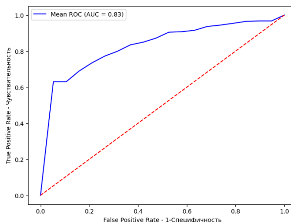
Рис.1. ROC-кривая модели классификации рамановских спектров злокачественной меланомы и себорейного кератоза методом логистической регрессии
