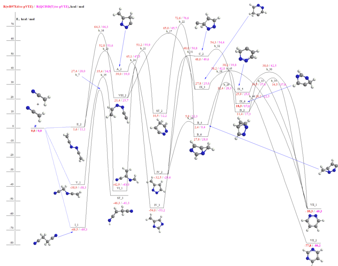
Рис. 1. ППЭ \text{CH}_2\text{CN} + \text{CH}_2\text{CN}
